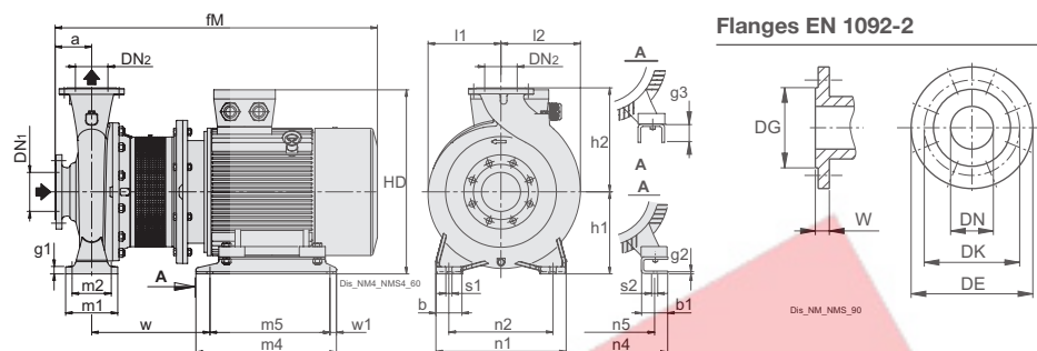
Flanges EN 1092-2
