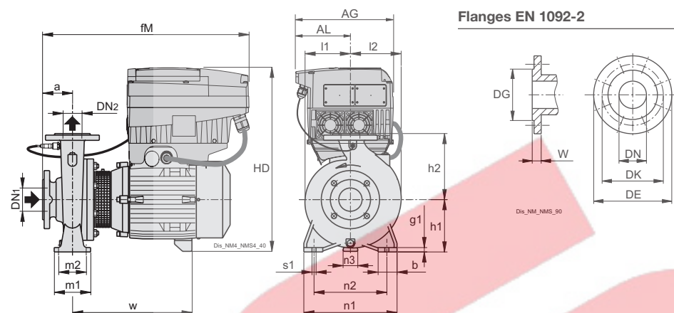
Flanges EN 1092-2
