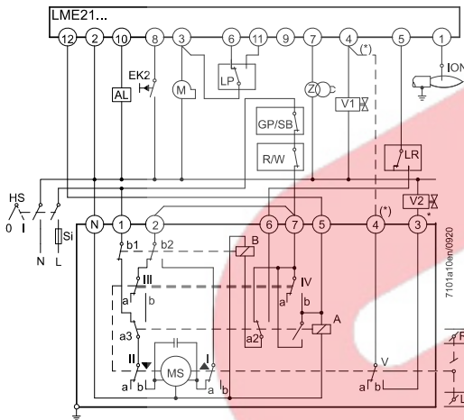
SQN3...121.../control de 2 etapas
