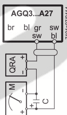
Medición realizada en el detector QRA...
