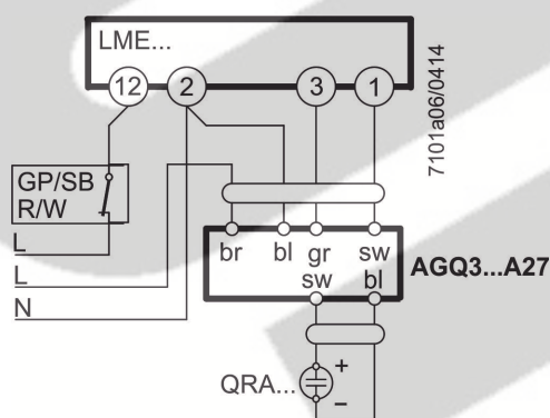
Diagrama de conexión
