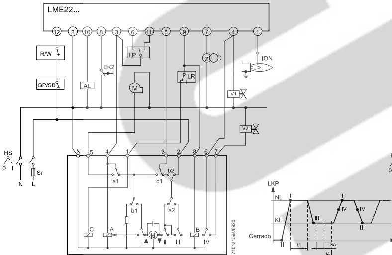
SQN7...454/control de 2 etapas control monofilar
