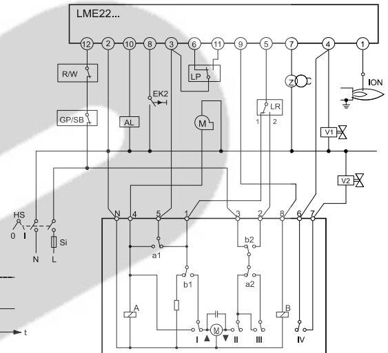
SQN7...424/control de 2 etapas control bifilar
