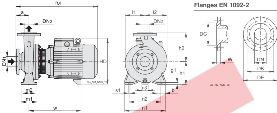
Flanges EN 1092-2
