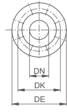
Flanges EN 1092-2
