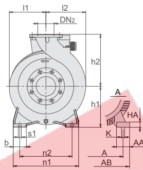
Flanges EN 1092-2
