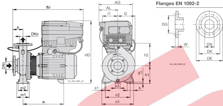
Flanges EN 1092-2
