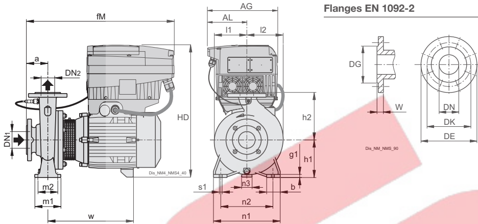
Flanges EN 1092-2
